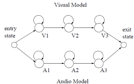
Şekil-1 : MSHMM topolojisi
