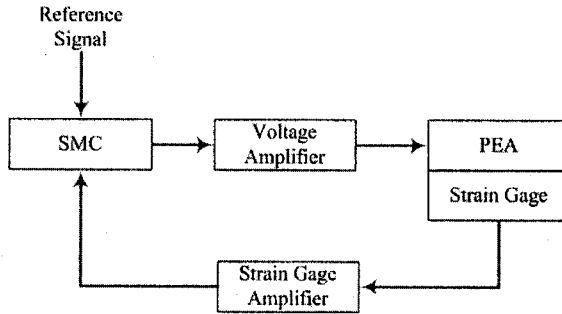
Fig. 5. Piezoelectric actuator control setup
