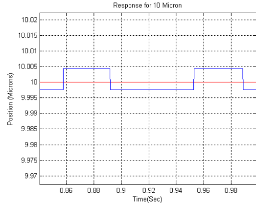
Şekil 7: Tasarım Çözünürlüğü (Bir kodlayıcı darbesi).
